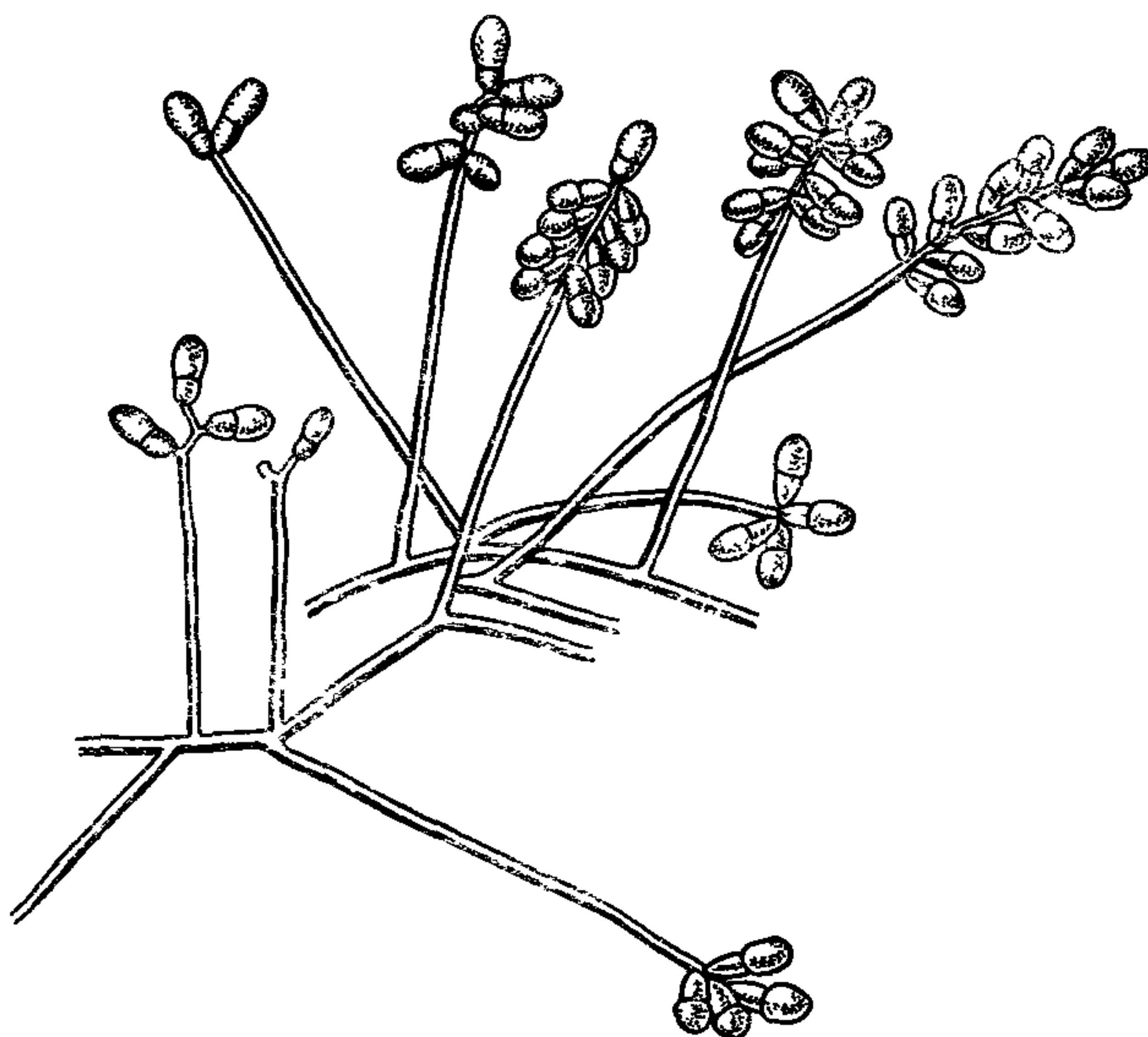
Конидиеносцы с конидиями Черт. 10
