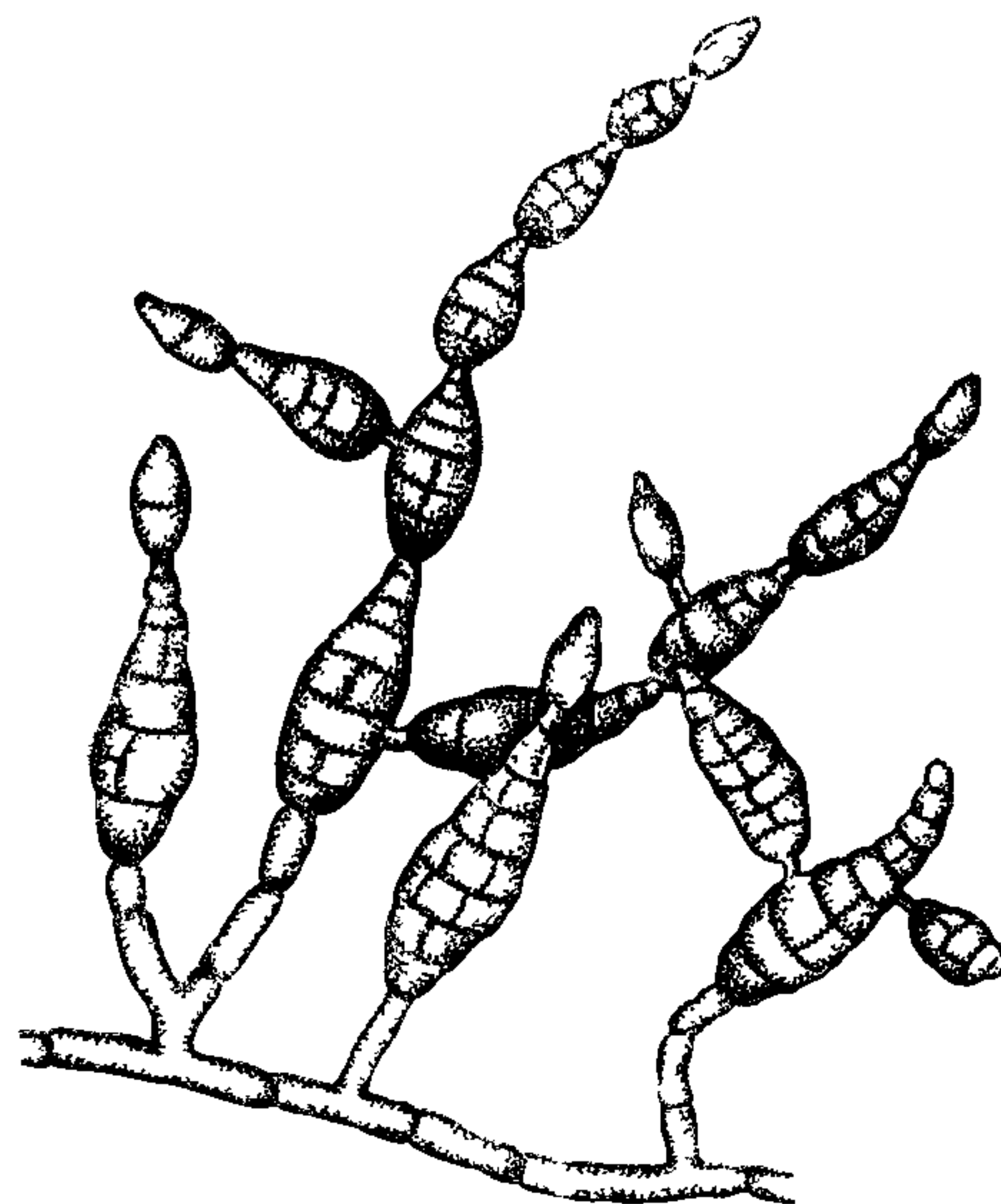
Конидиеносцы с цепочками конидий
