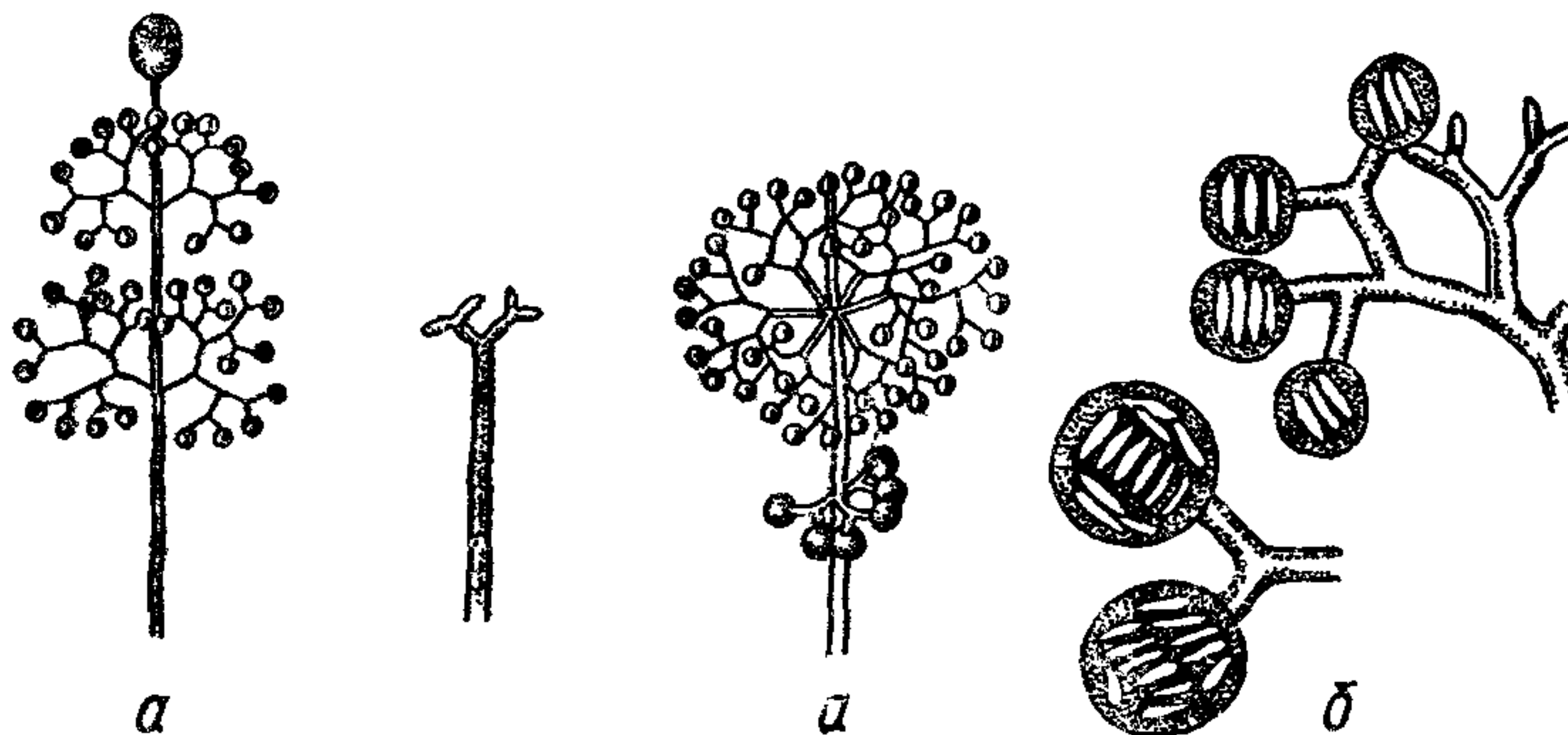
Спорангиеносец со спорангиями (спорангиолями) а—при малом увеличе нии, б—при большом увеличении
