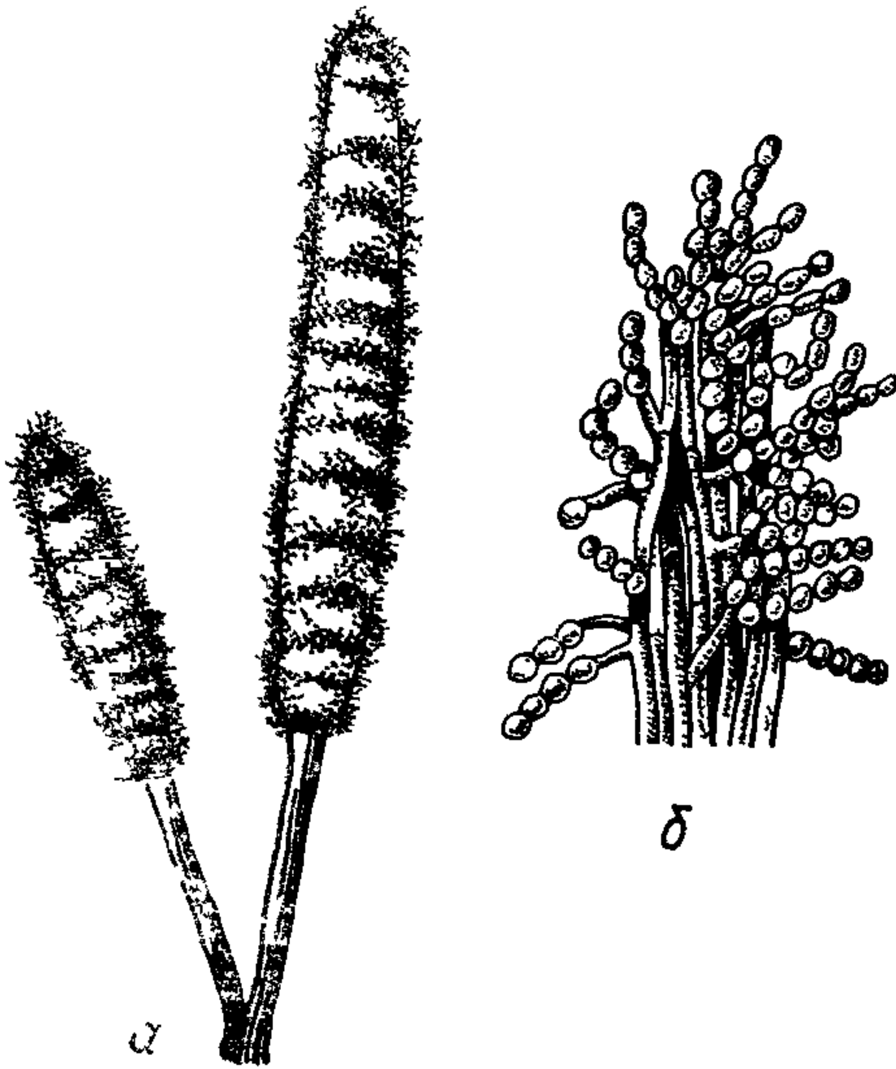
Коремки с конидиями а—при малом увеличении, б—при большом увеличении
