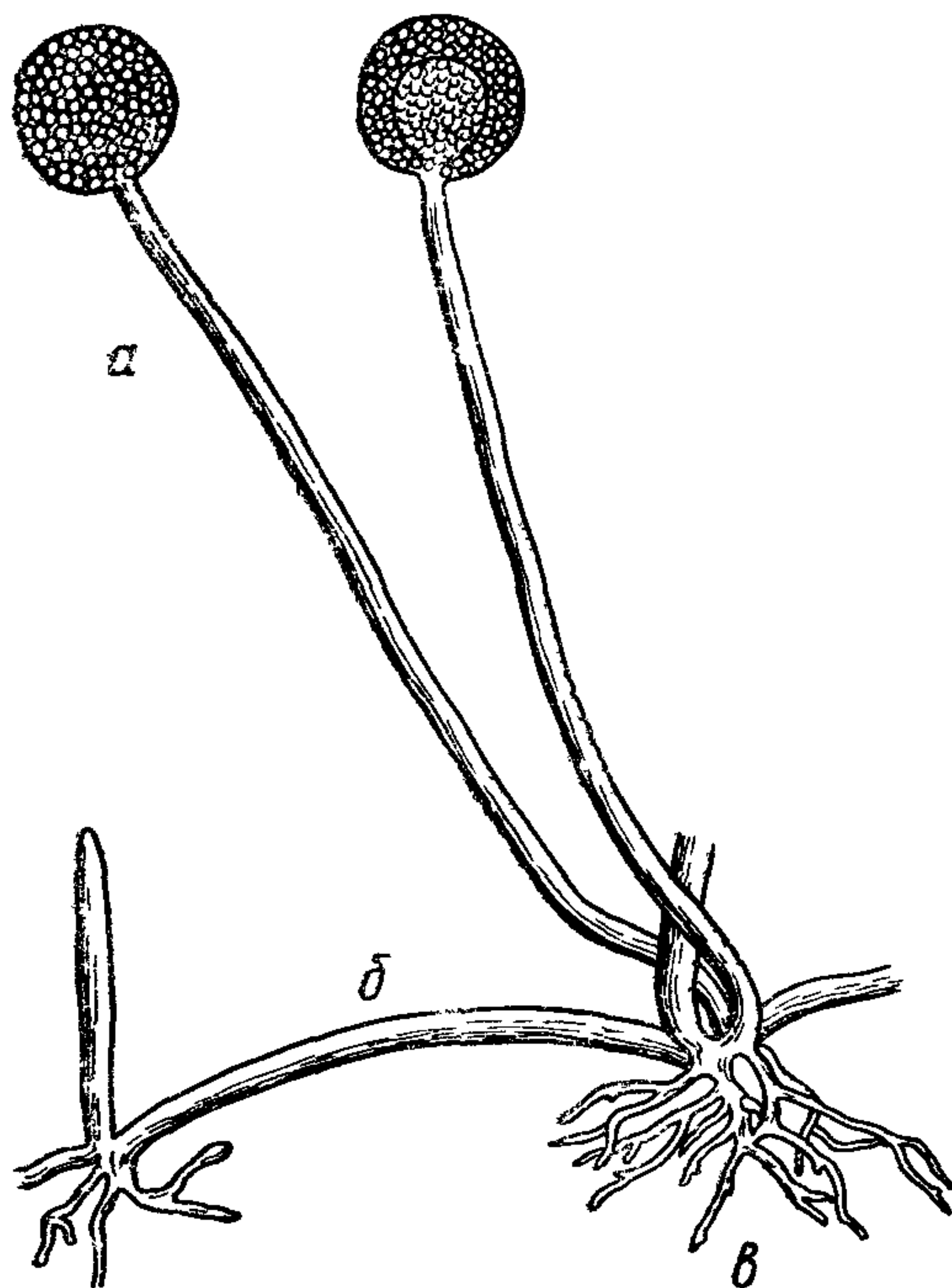
а—спорангиеносцы со спорангиями, б—столоны, в—ризиды.
