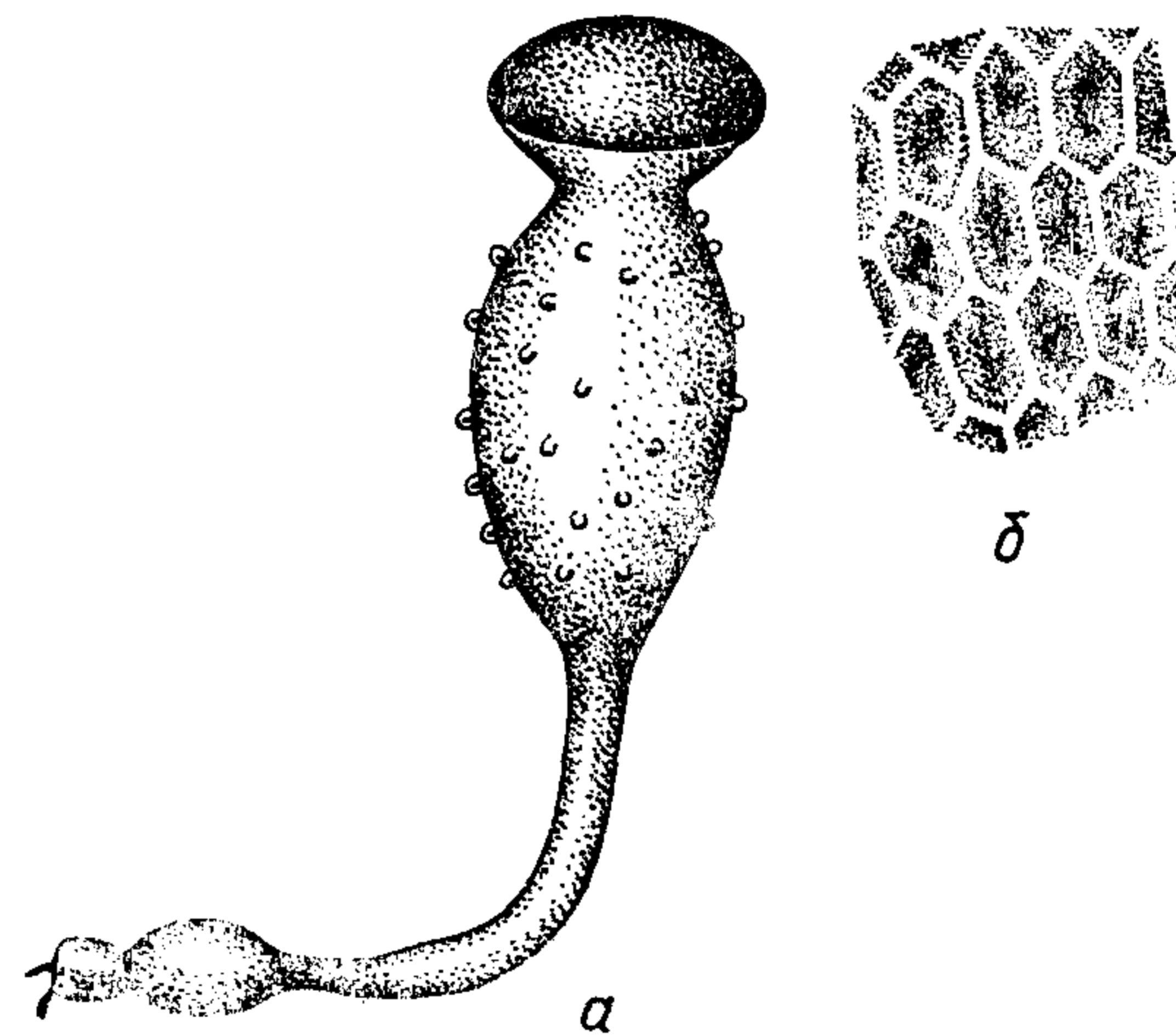
a —спорангиеносец; б —оболочка спорангия
