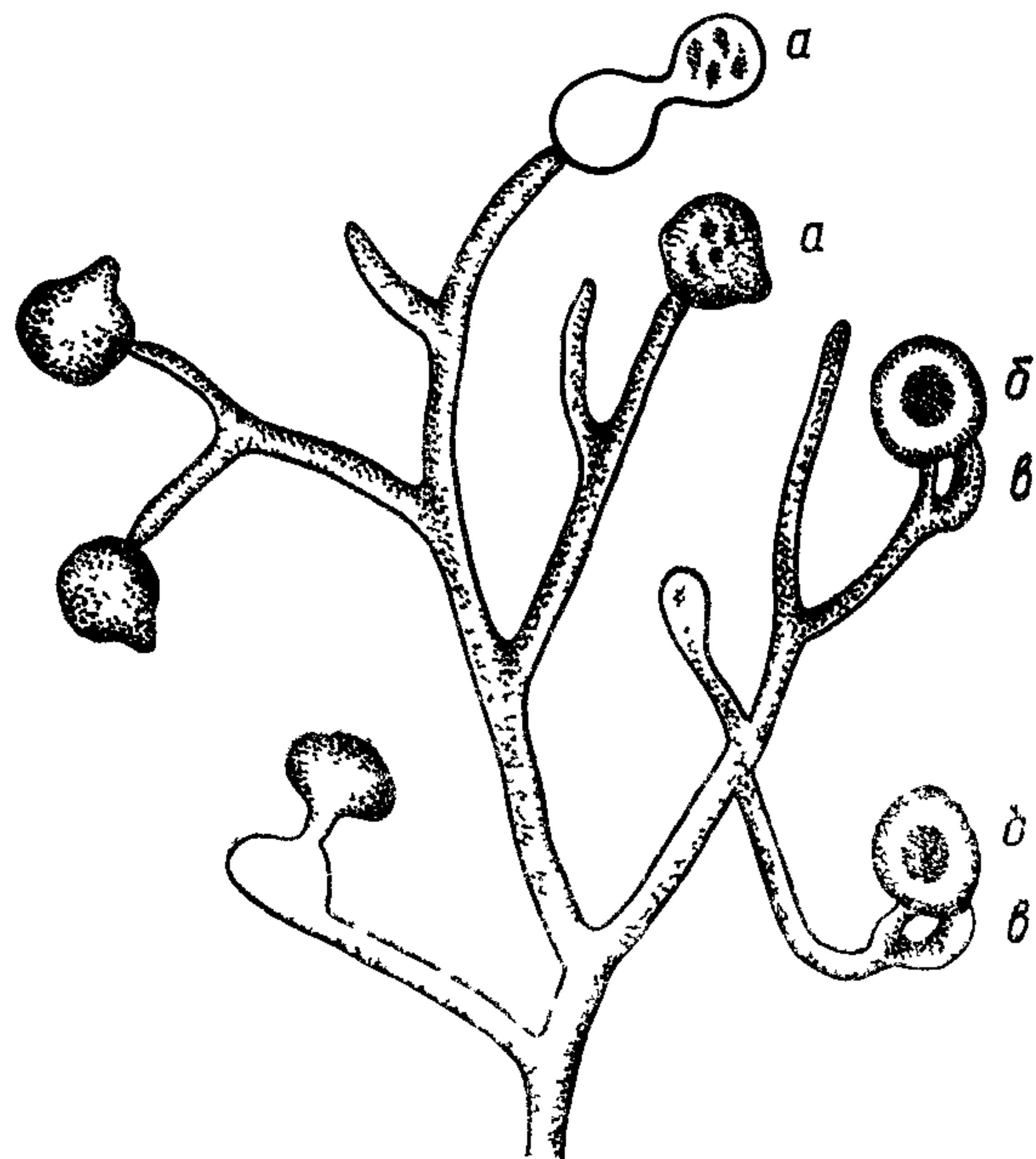
а зооспорангий, б ооспора в антеридий
