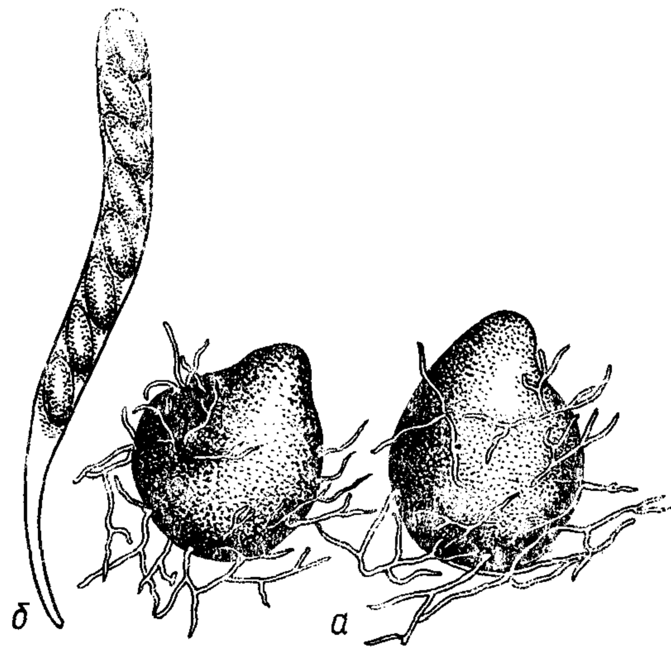
a —перитеций; б —сумка с аскоспорами
