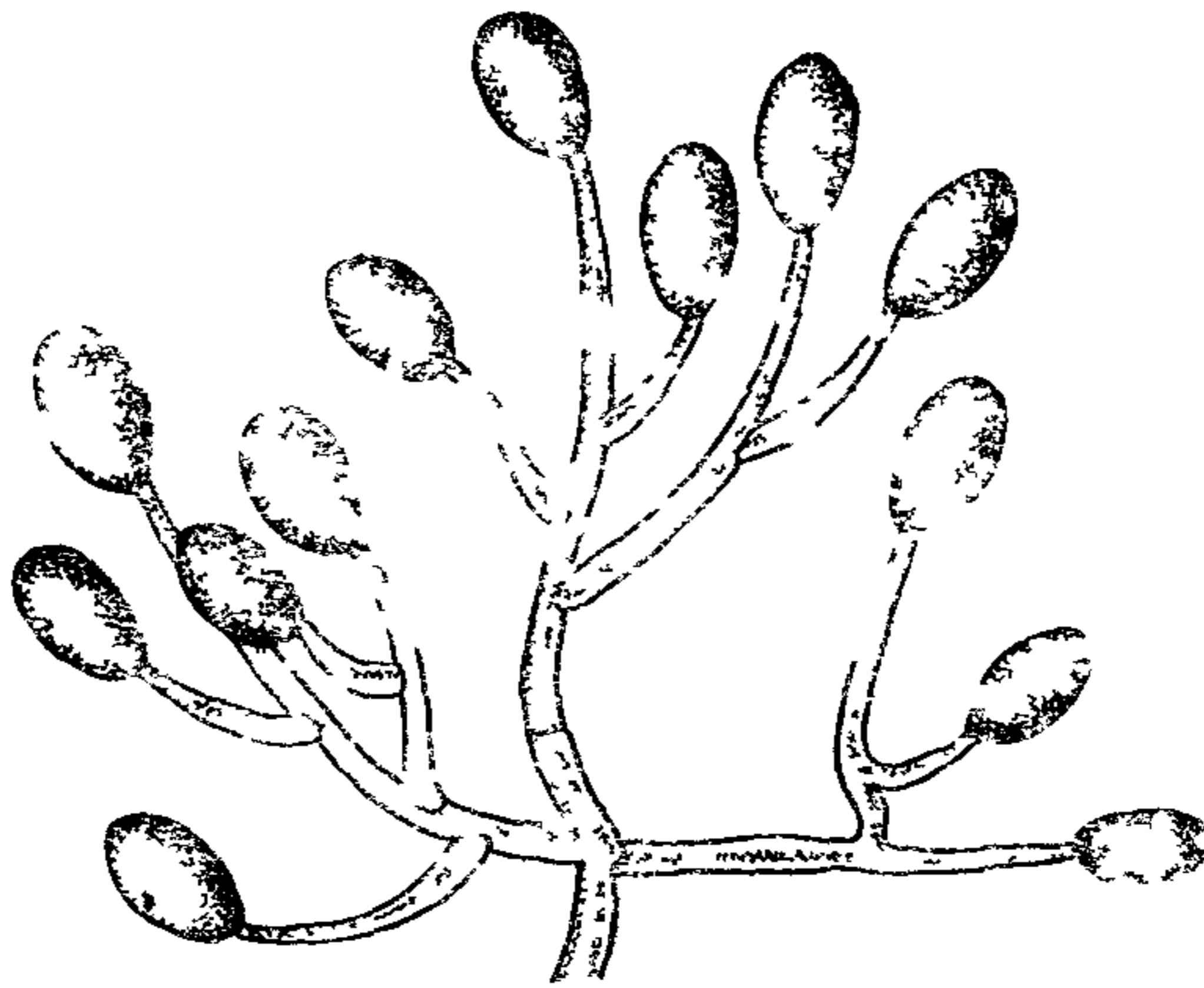
Конидиеносец с одиночными конидиями Черт. 3
