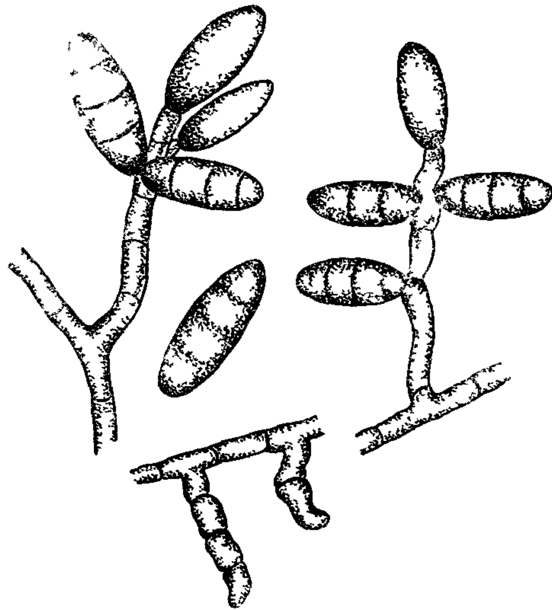
Конидиеносцы с конидиями
