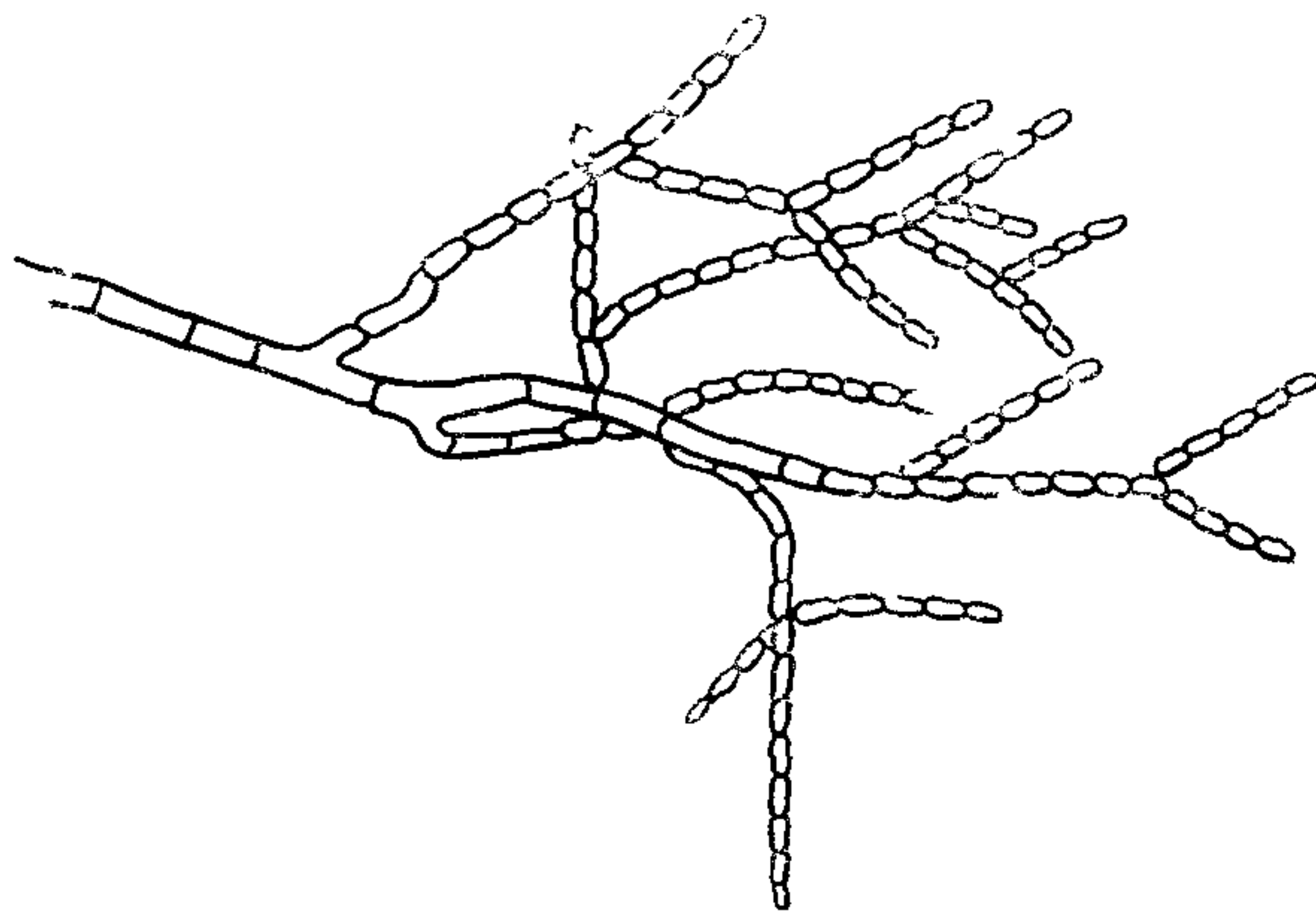
Конидиеносцы с цепочками конидий Черт. 9
