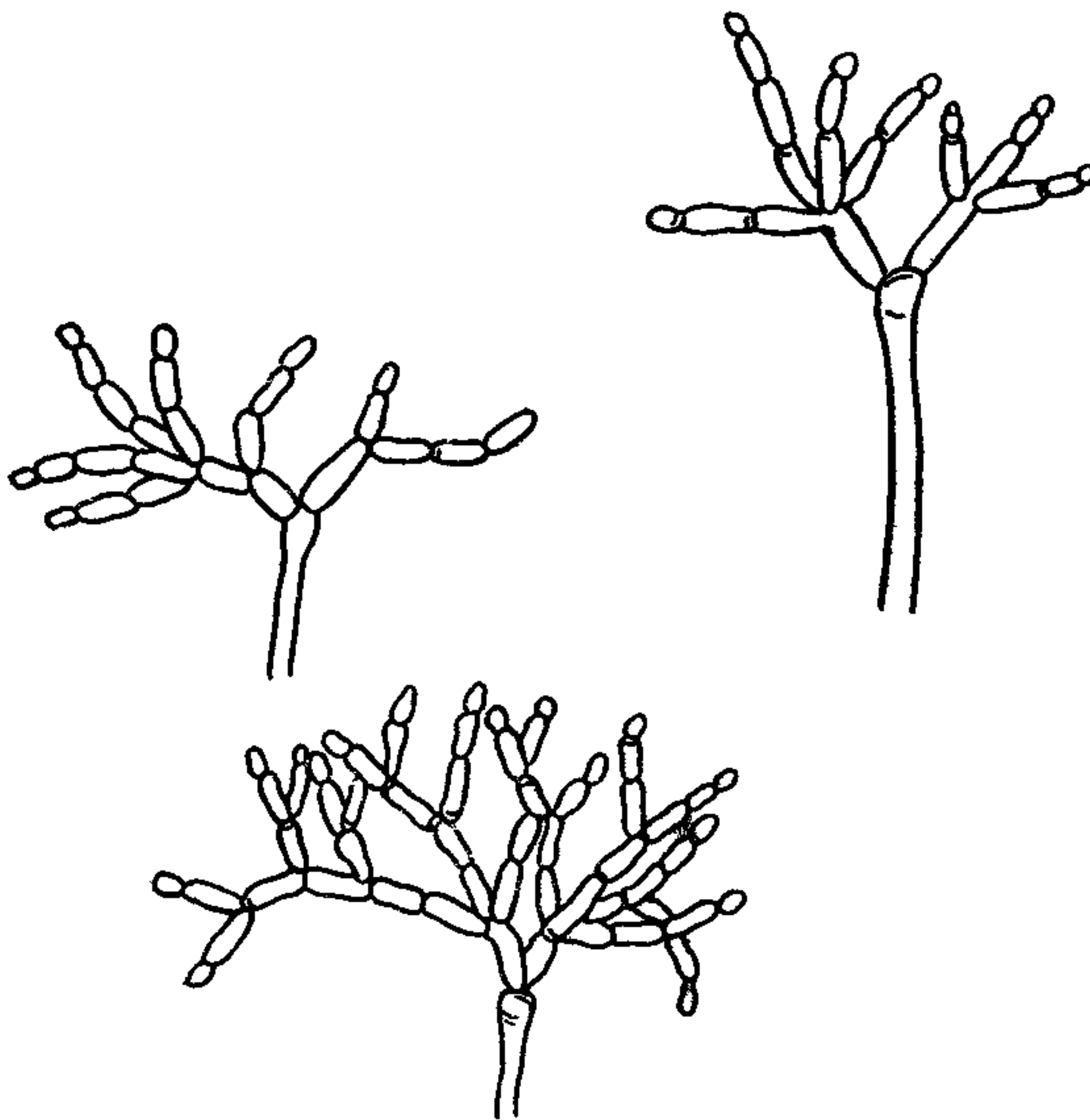
Конидиеносцы с конидиями
